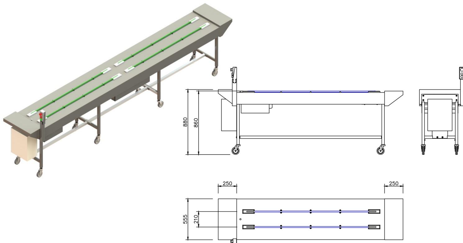
Convoyeur servant à la préparation de plateaux repas.
