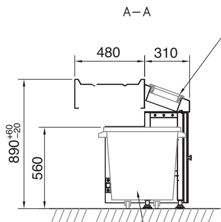
1 poubelle plastique sur socle rouleur par TVO 1 dustbin, on wheels, per scrapping ring
