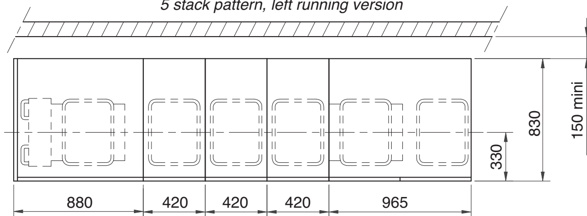
Modèle 5 piles gauche-droite 5 stack pattern, left running version
