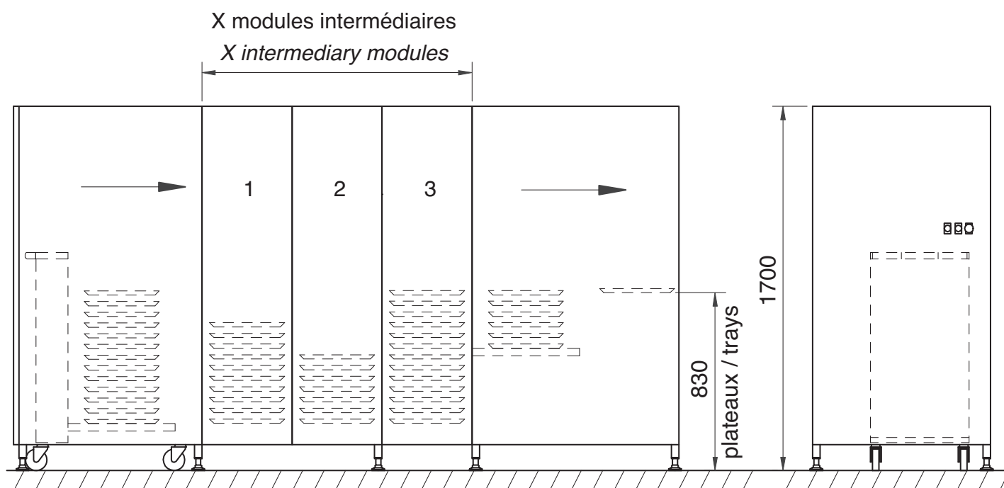
Modèle 5 piles gauche-droite 5 stack pattern, left running version
